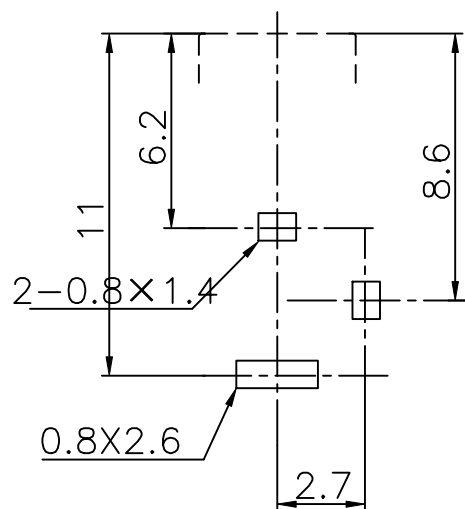
线路板开孔尺寸
