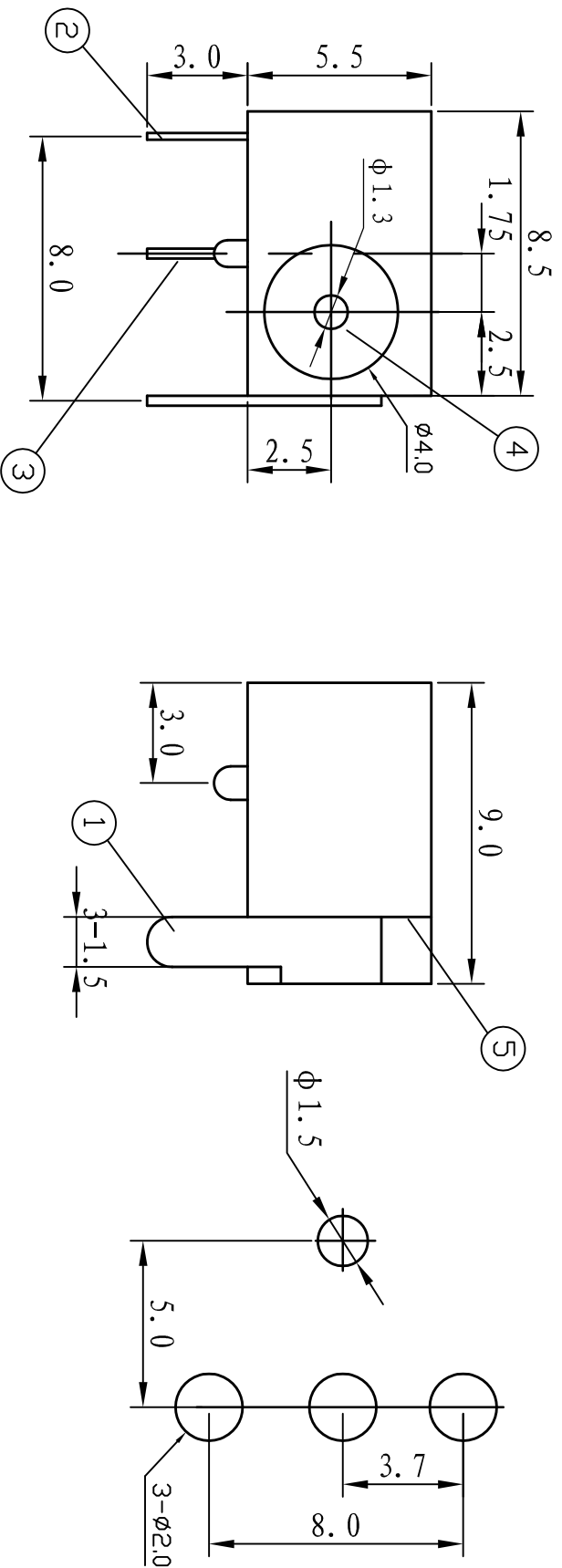
线路板安装尺寸示意图
