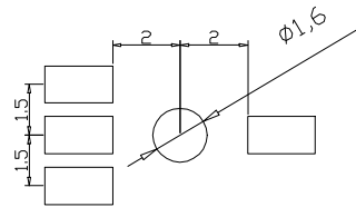
安装尺寸
