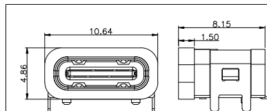
加防水圈示意图
