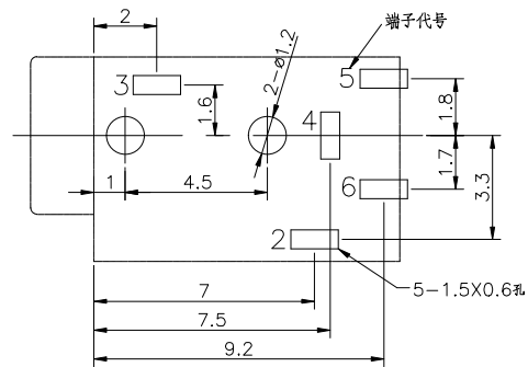
PCB, 开孔尺寸图 Top View
