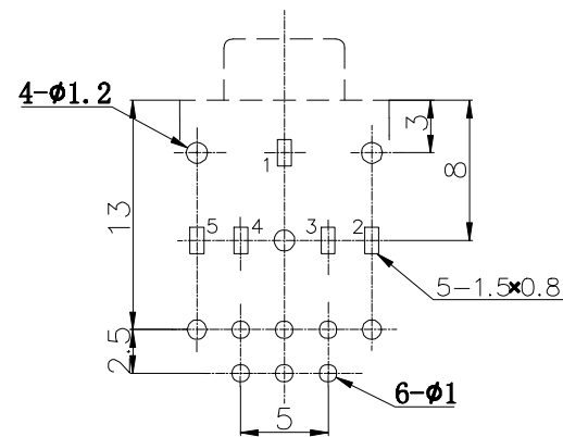
线路板开孔尺寸
