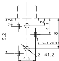
线路板开孔尺寸
