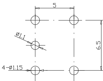
安装尺寸
