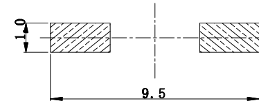
P.C.B LAYOUT
