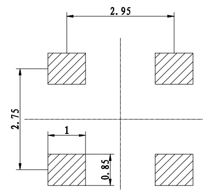
P.C.B LAYOUT
