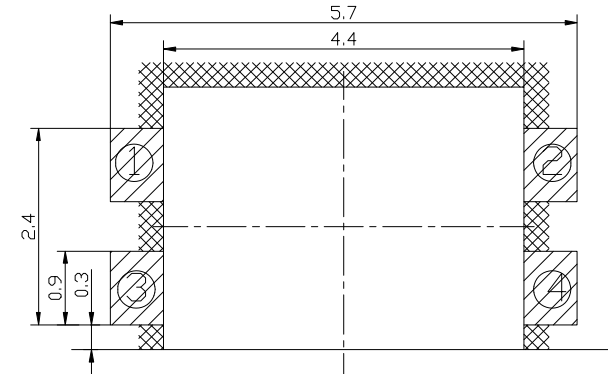
安装参考图
